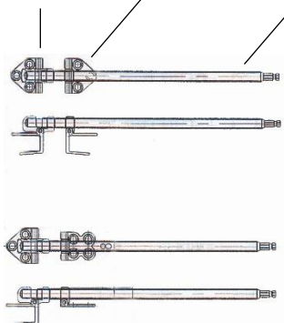
固定用プレート、移動用プレート、シャフト
