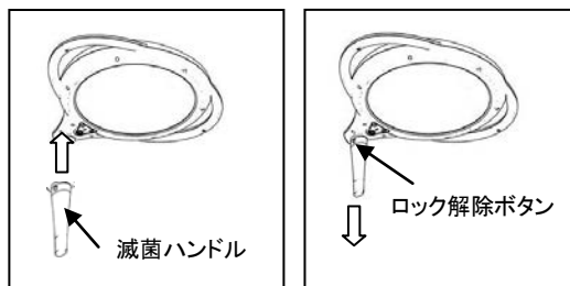
【取り付け方法】
