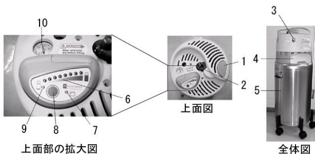
図 2 設置用容器（ヘリオス 36/ヘリオス 46）
