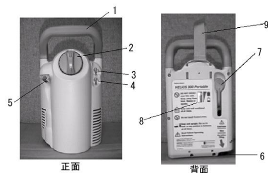
図 1 携帯用容器（ヘリオス 300）
