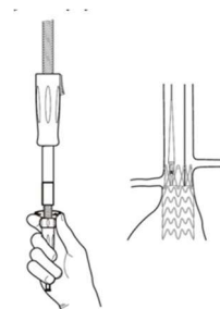
図 A7 テーパ状チップ内へのスピンドル再格納
