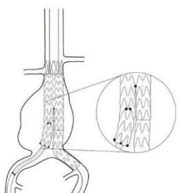
図 B10 イリアックデリバリーシステムの挿入 - ステント 3 個分の重複
