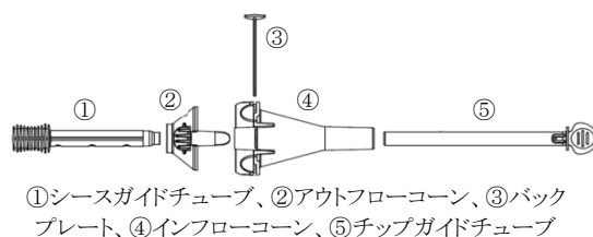
図 3 装填システム(LS)
