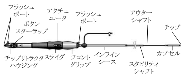
図 2 デリバリーカテーテルシステム(DCS)
