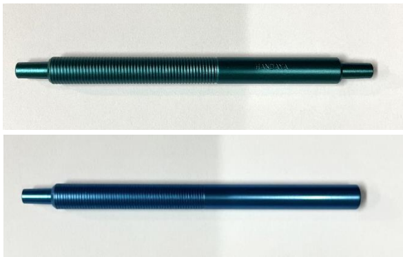
上 : バイマニユアルハンドピース 吸引 ハンドルのみ 下 : バイマニユアルハンドピース 灌流 ハンドルのみ 材質 : アルミニウム 眼科手術時に吸引/灌流に用いるカニューレを取付けるハンドル。
