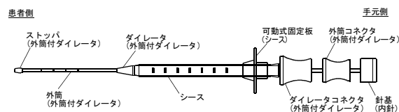
外観図
