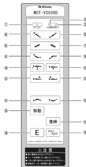
図 6-1 : 操作ボックス (18-600-10・18-610-10 用)
