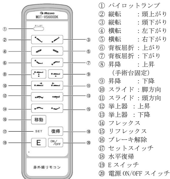
図 7-2 : コードレス操作ボックス (18-043-56)
