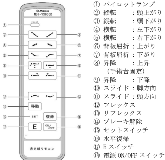
図 7-1 : コードレス操作ボックス (18-043-53)
