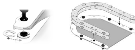
(シム使用例) (SRS 用シングルシム使用例)
