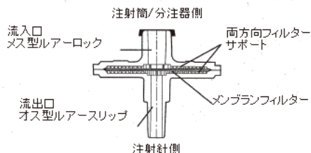
構造図
