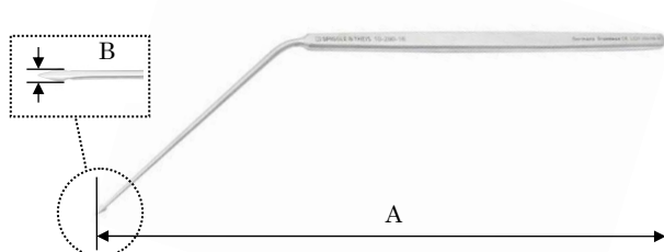
① S & T P o l i t z e r 式鼓膜パーフォレーター **
