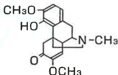
sinomenine
