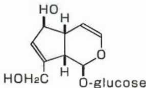
aucubin
