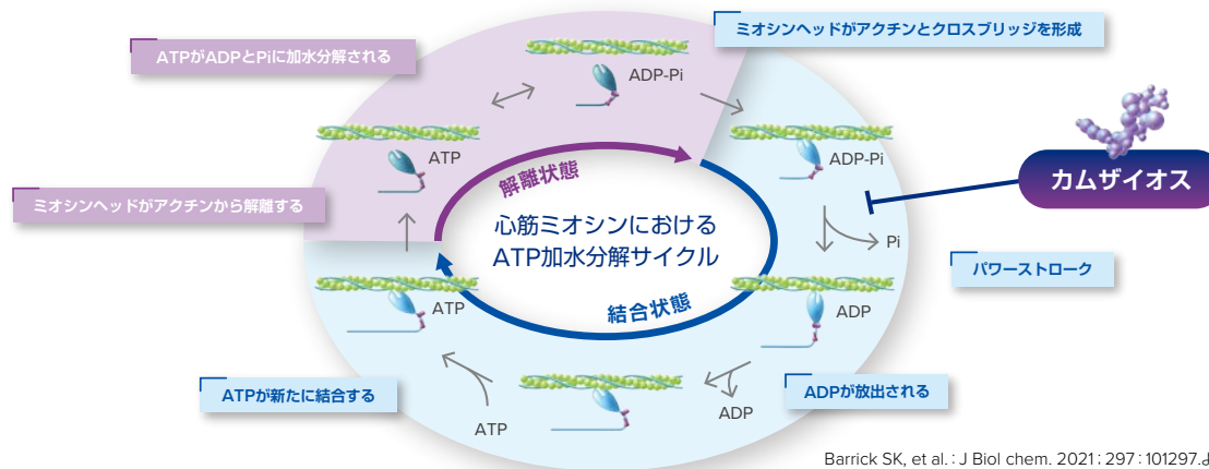
図2 ATP加水分解サイクルにおけるマバカムテンの作用 2),3)
