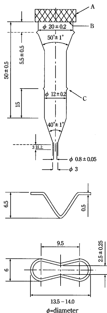
Fig. 6.10-4 Apparatus 3
