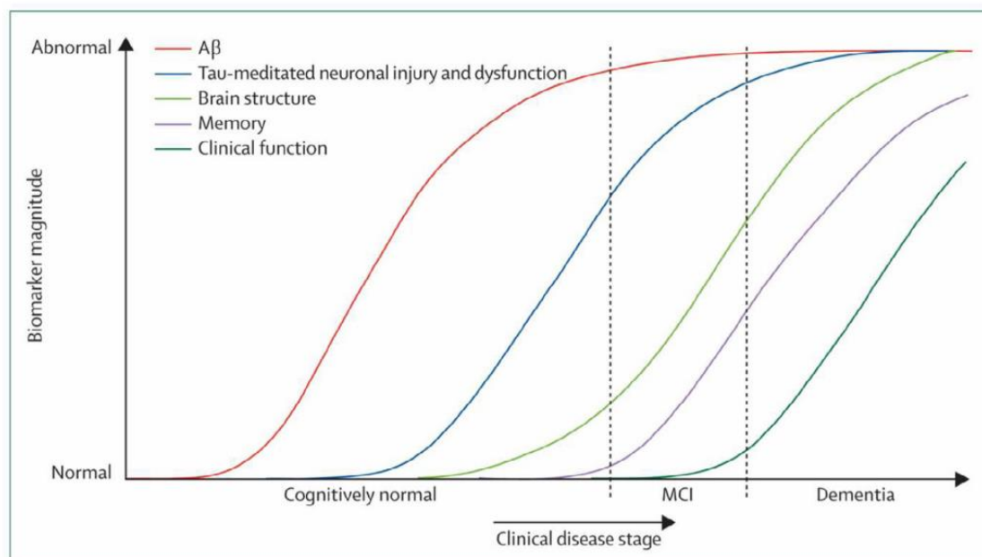
図2：ADの発症に至るバイオマーカーの推移（Jack et al. Lancet Neurol 2010 より引用） 60)
