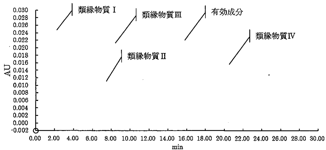
図*** 類縁物質の各クロマトグラム
