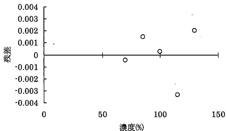
図*** (5) 定量法 残差プロット
