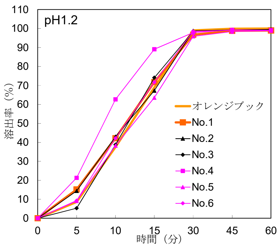
図 57 オフロキサシン錠 100mg の pH1.2 における溶出挙動
