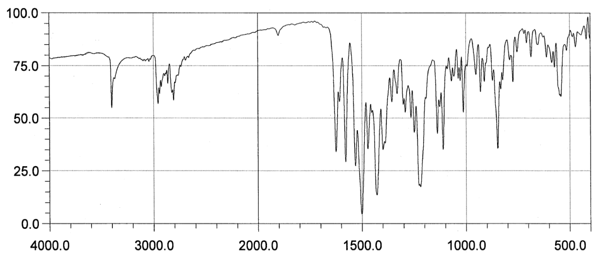
Gefitinib
