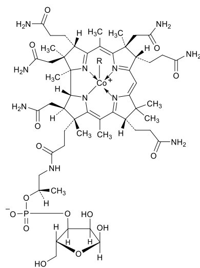
40 cobamide
