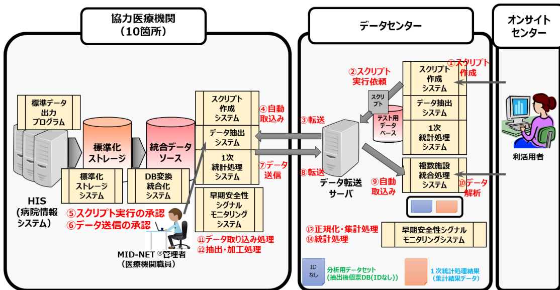
図 4 利活用に関係する主な処理
