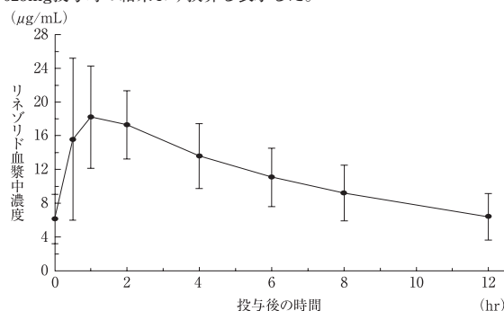
図1 リネゾリド600mgを1日2回12時間ごとに反復経口投与した後の定常状態における血漿中濃度推移(Mean ± S.D.、外国人、n=16)
