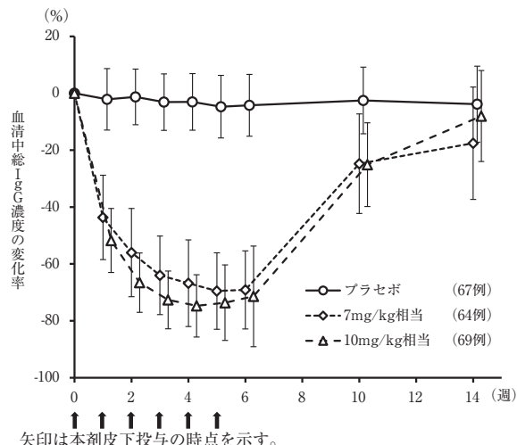
図2 血清中総IgG濃度のベースラインからの平均変化率(±標準偏差) (MG0003試験：Safety Set)
